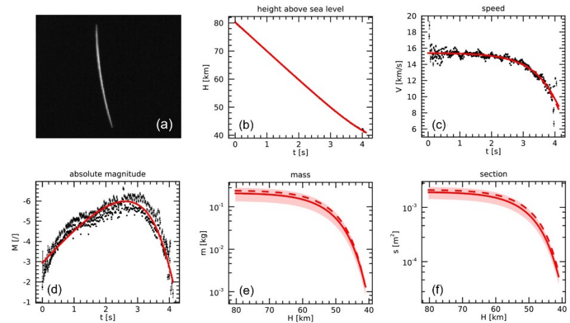
Meteorite «Cavezzo»
