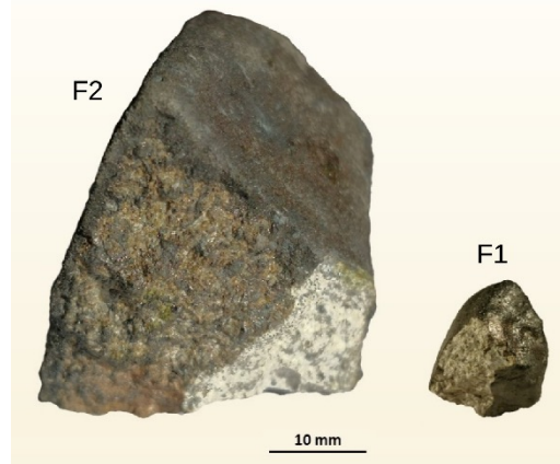
Meteorite «Cavezzo»
