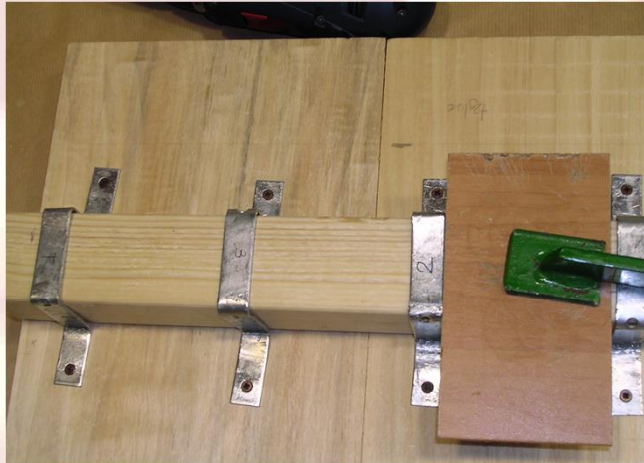
Traverse con ponticelli metallici
